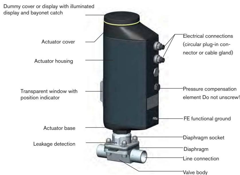
Aufbau, elektromotorisches Membran-Regelventil Typ 3323
